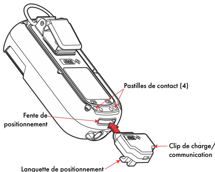
Figure 49 : Connexion du clip de charge/communications
