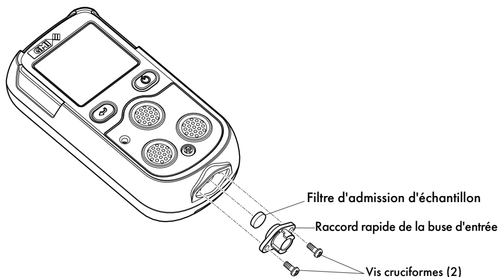
Figure 53 : Remplacement du filtre (poussière) d'admission d'échantillon
