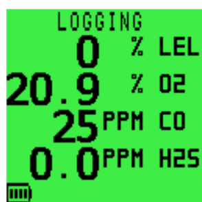
Figure 20 : Sauvegarde manuelle
