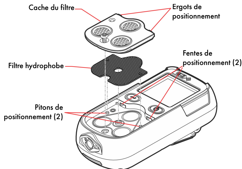
Figure 52 : Remplacement du filtre hydrophobe
