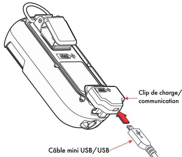
Figure 50 : Connecter le câble au clip de charge/communications
